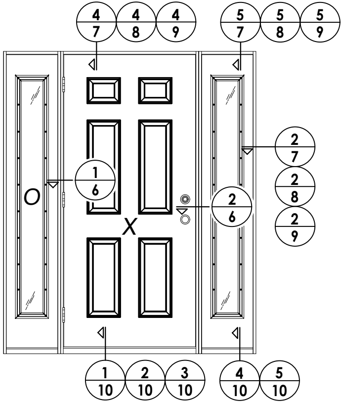
ELEVATION OXO
